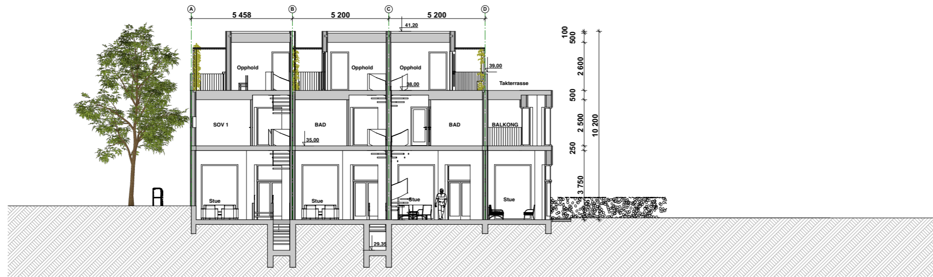
SNITT A-A
