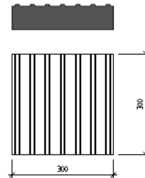
Detalj retningsindikator
