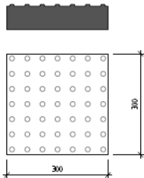
Detalj varselindikator
