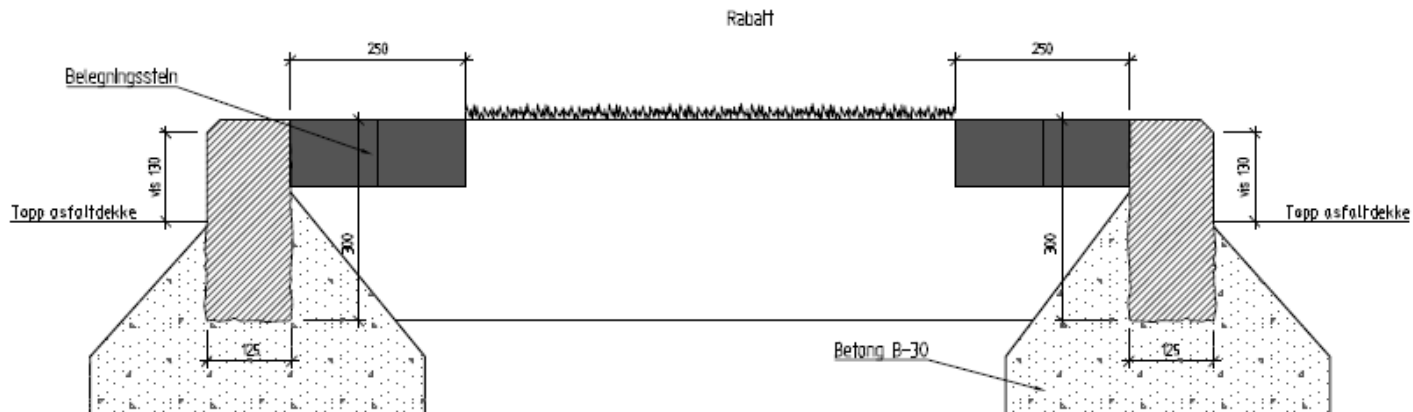
Kantstein busslomme
