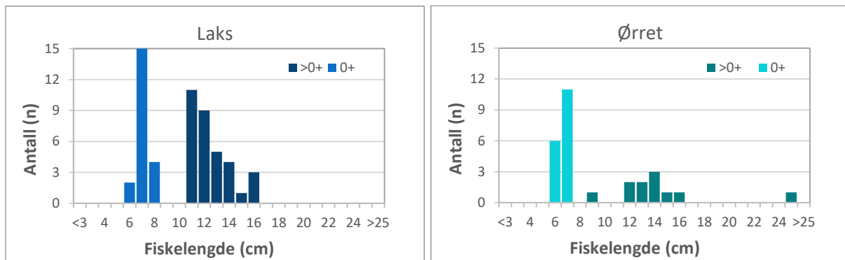
Figur 50. Lengdefordeling for laks (venstre) ørret (høyre) på fem elektrofiskestasjoner i Høleåna (se kart i Figur 22 og Figur 49 ). Elektrofisket ble utført 15. november 2022.
