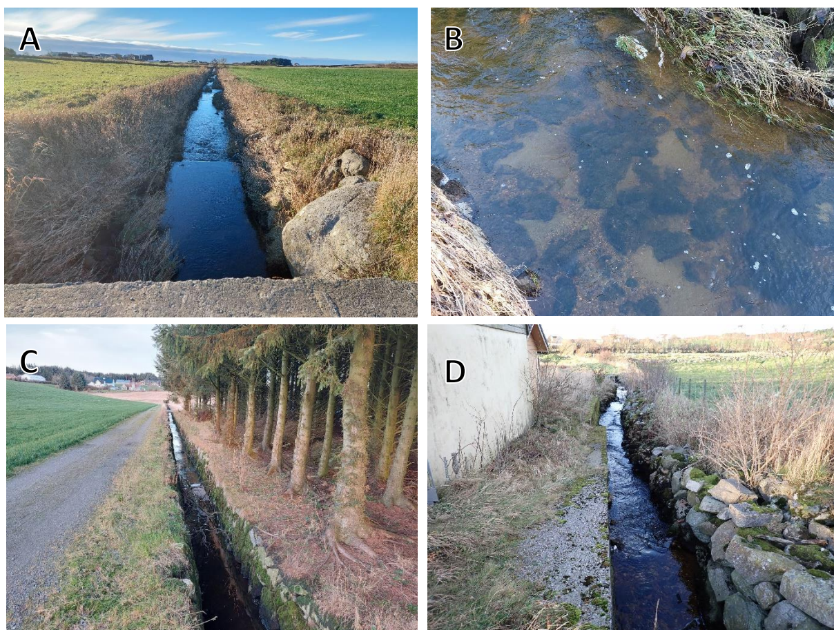
Figur 6. Morfologiske inngrep i Hørråna: A) Kanalisert elveløp og manglende naturlig kantvegetasjon B) Mye finstoff er akkumulert på bunnen C) Utrette og forbygd strekning med manglende kantvegetasjon D) kanalisert og utrettet strekning i sideløpet (segment 53).
