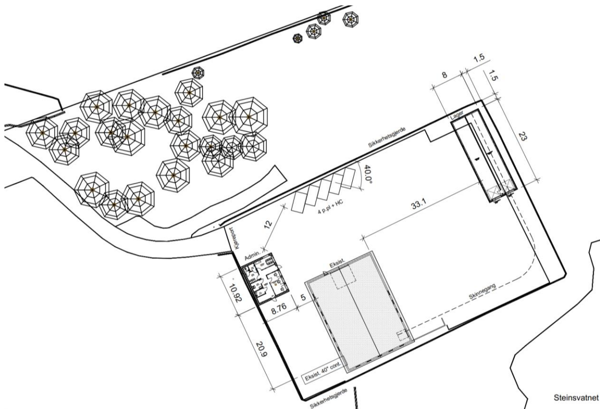
Figur 2.2: Situasjonskart som viser mulig nytt administrasjonsbygg med garerobefasiliteter til venstre og nytt lagerbygg oppe til høyre.
