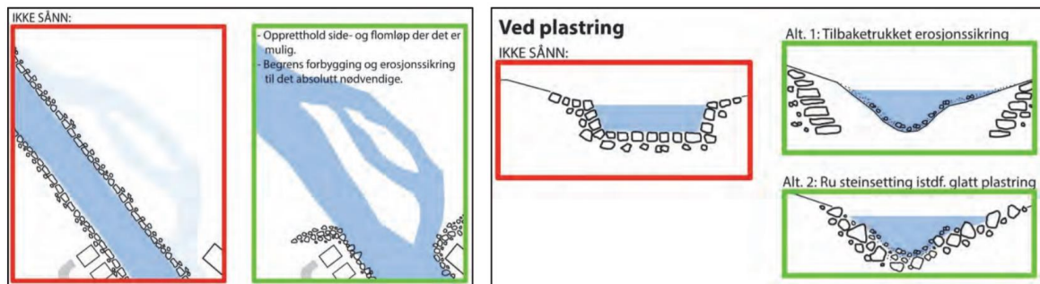
Figur 2. Prinsippskisse for miljøvennlig erosjonssikring. Rødt: nei, grønt: ja. Gjengitt fra Miljødirektoratets tiltakshåndbok for bedre fysisk vannmiljø (Pulg, et al., 2018).
