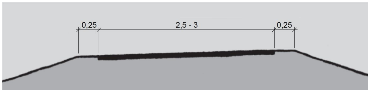
Figur 17: Tverrprofil på gang- og sykkelveg med skuldre. Hentet fra Statens vegvesens håndbok N100 figur 4.2.1.1-1.
