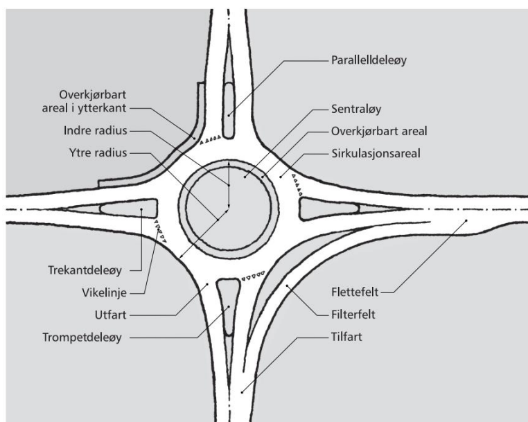
Figur 4-12: Ulike elementer i en rundkjøring. Kilde: Håndbok V121
